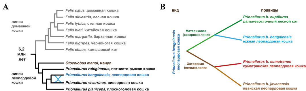
Рис. 1. А – сестринские линии домашней и леопардовой кошки, выявленные в ходе исследований митохондриальных и ядерных геномных участков (Johnson et al. 2006); В – генетически различные подвины леопардовой кошки P. bengalensis , выявленные в ходе генетических исследований (Luo et al. 2014; Patel et al. 2017).
